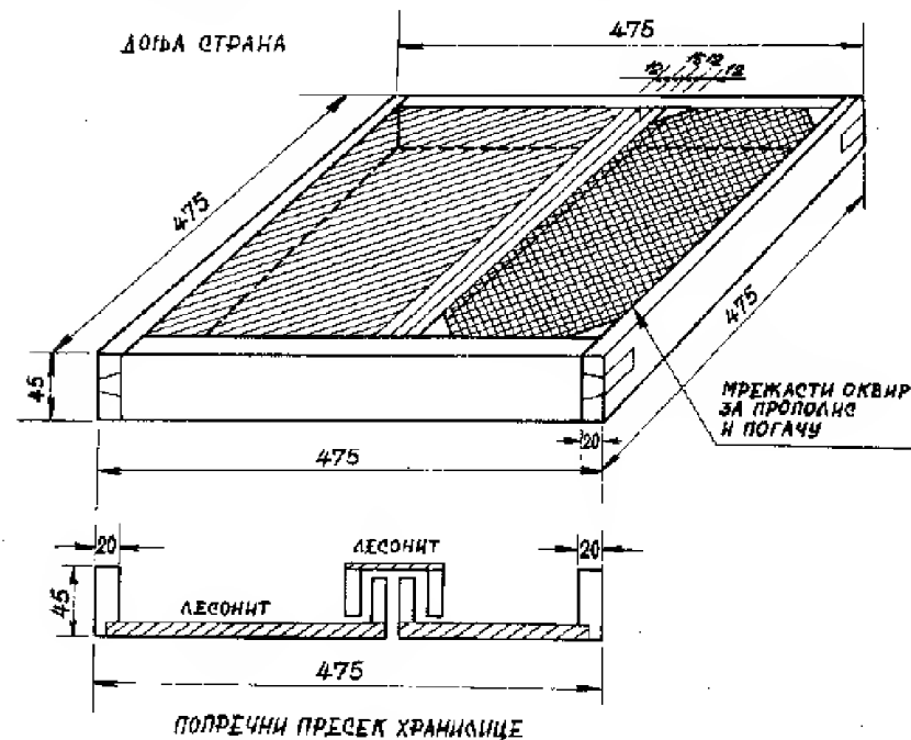
Хранилица др Милера са допуном оквира за прикупљање прополиса горња страна
